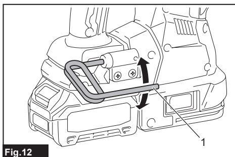
Fig.12 ► 1. Crochet
