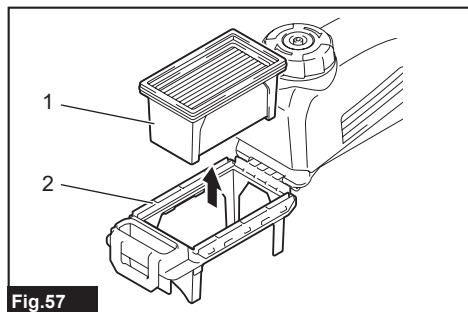
► 1. Filtre 2. Boîtier de filtre
