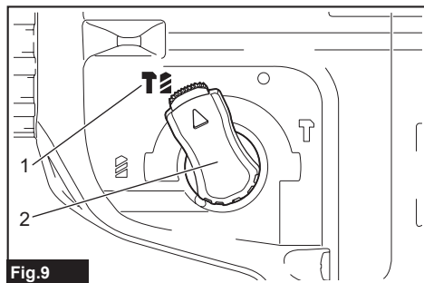
Fig.9 ► 1. Rotation avec percussion 2. Bouton de changement de mode
