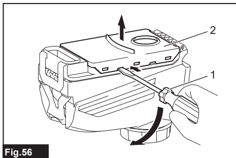
► 1. Tournevis à lame plate 2. Couvercle de filtre
